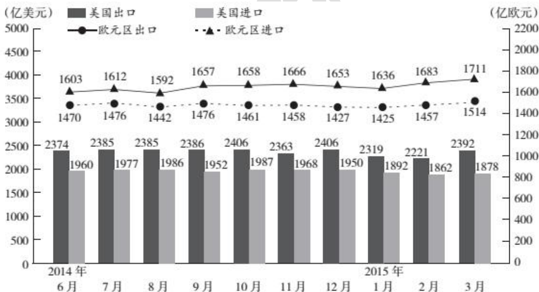
图 2014 年 6 月~2015 年 3 月美国与欧元区进、出口额
